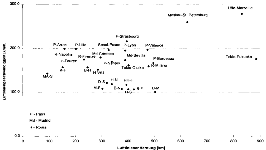
Abbildung 9 59)60) : Leistungsvergleich von Hochgeschwindigkeitssystemen verschiedener Länder
