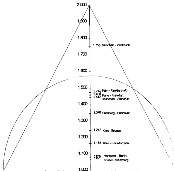
Abbildung 8 53) : Umwegfaktor Diagramm
